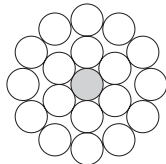
18 Al - 1 Aço 18 Al - 1 Steel
