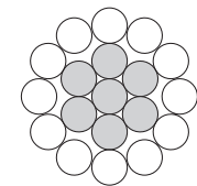
12 Al - 7 Aço 12 Al - 7 Steel
