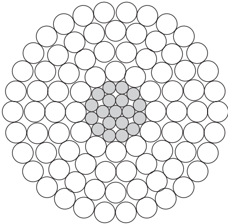
84 Al - 19 Aço 84 Al - 19 Steel
