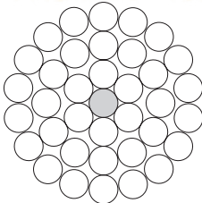
36 Al - 1 Aço 36 Al - 1 Steel
