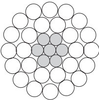
26 Al - 7 Aço 26 Al - 7 Steel
