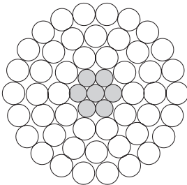
45 Al - 7 Aço 45 Al - 7 Steel
