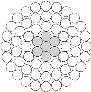
54 Al - 7 Aço 54 Al - 7 Steel
