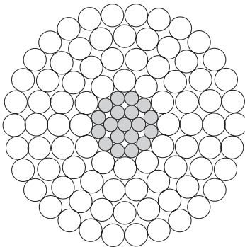
84 Al - 19 Aço 84 Al - 19 Steel
