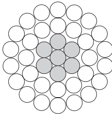
30 Al - 7 Aço 30 Al - 7 Steel
