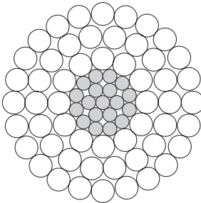
54 Al - 19 Aço 54 Al - 19 Steel
