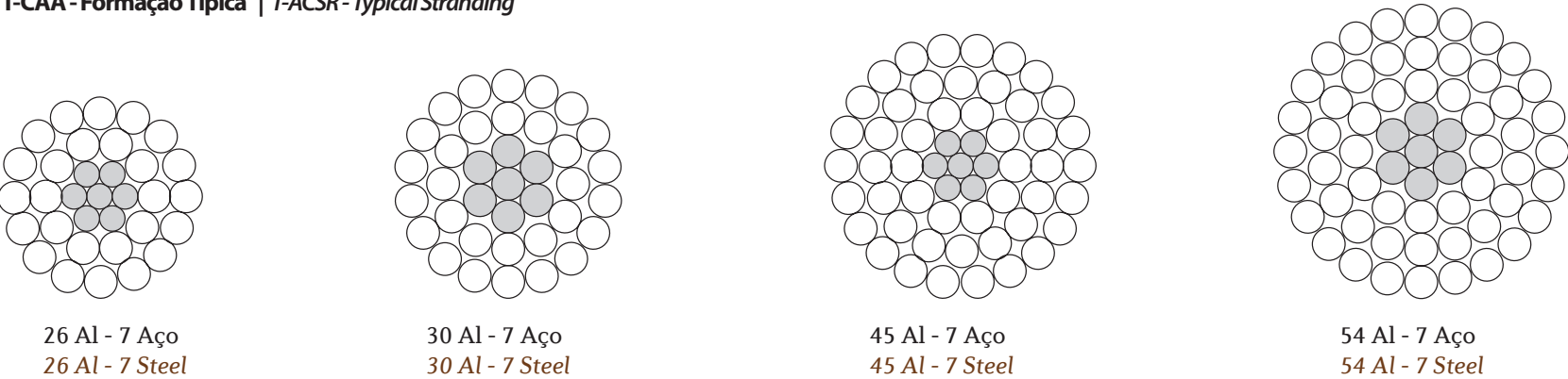
T-CAA - Formação Típica | T-ACSR - Typical Stranding
